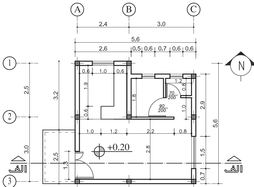
پلان طبقه همکف
