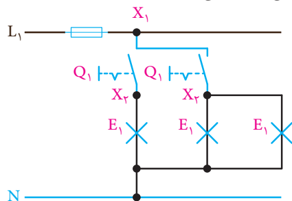
شکل ۳۱- نقشه گسترده مدار کلید دابل
