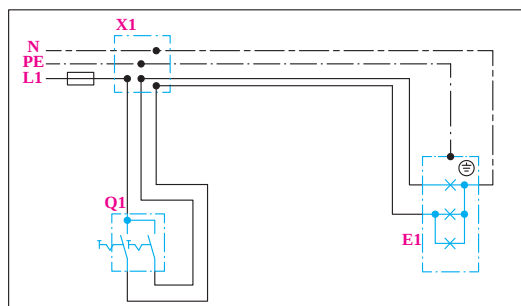
شکل ۲۹- شمای حقیقی مدار کلید دابل
