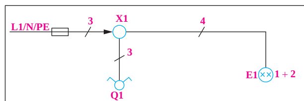
شکل ۳۰- شمای فنی مدار کلید دابل
