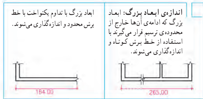
شکل ۱۵-۴- روش های اندازه گذاری
