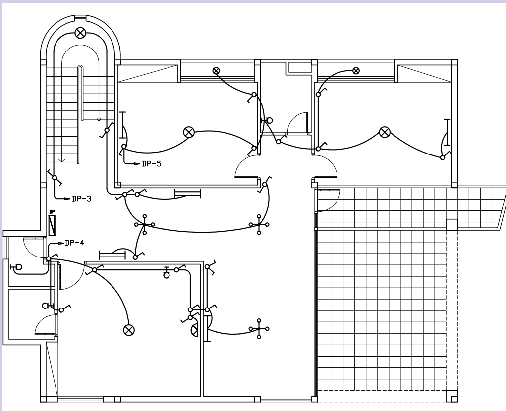
شکل ۳-۷۴- پلان روشنایی و پریرز
