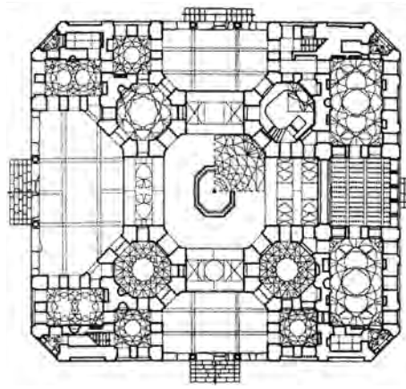
پلان طبقه اول
