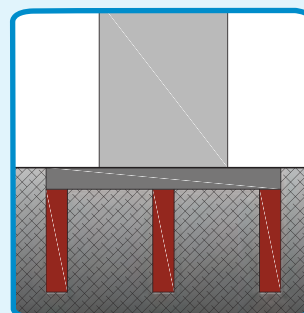
شکل ۱۷-۲- گروه شمع‌ها
